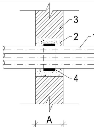
Fig. 5. Um feixe de tubos em uma parede
