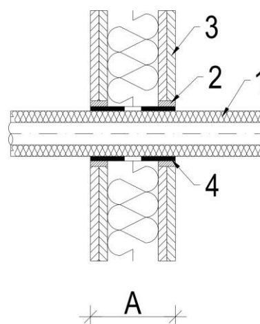
Fig. 8. Um único tubo com borracha em uma parede de gesso
