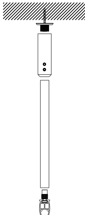
MTS Support de suspension au plafond
