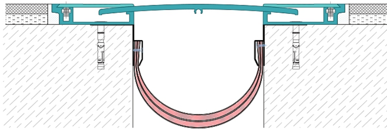
» Aplicação de barreira corta-fogo sob perfil de junta de dilatação / Fire barrier application under expansion joint profile
