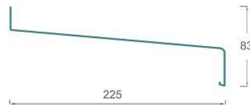
CCR052_606 25CM PARAPETO / PARAPET
