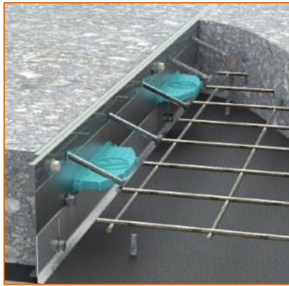
» JUSTO DESPUÉS DE VERTER EL CEMENTO RIGHT AFTER POURING CONCRETE
