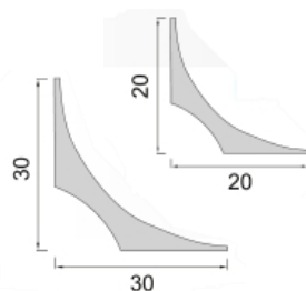
CPS28 Perfil de la tapa (puede ser producido en varios colores) Cap profile (can be produced in various colors)
