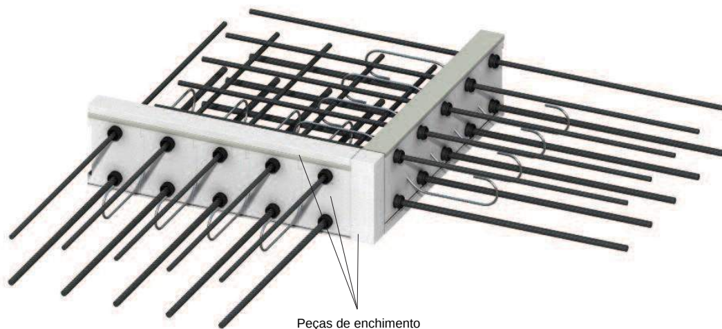
Detalhe de canto com Isolan
