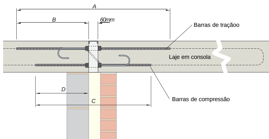
Comprimentos dos varões de reforço
