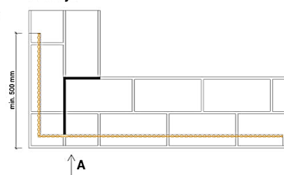
Půdorys
