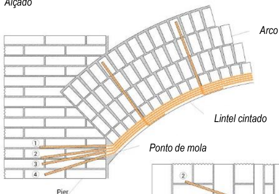
Alçado
