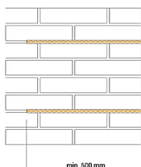
Pohled B
