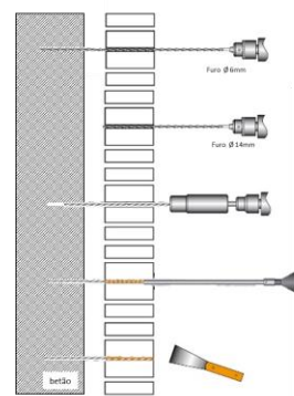
Aplicação de STATI-Tie em betão para fixação de alvenaria
