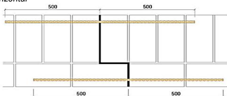
Corte Horizontal
