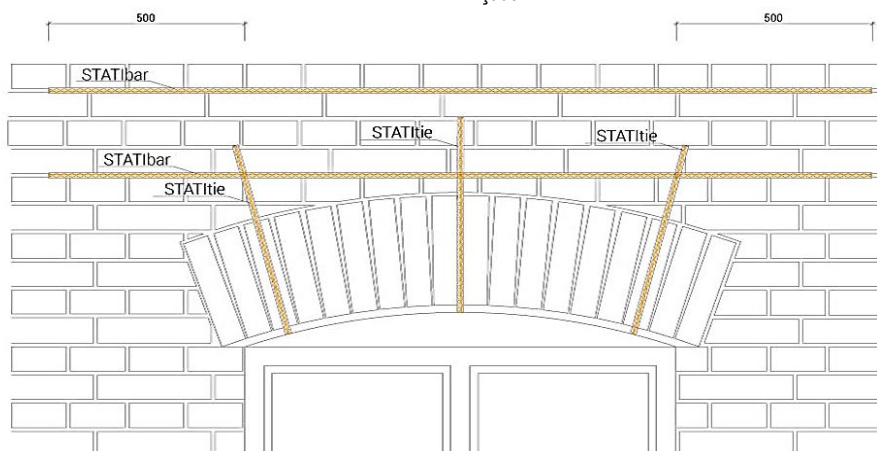
Alçado
