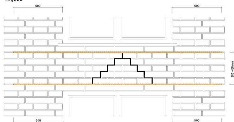
Alçado
