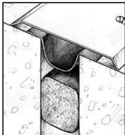
Bandade estanquicidade com cordão cortafogo e cobre-juntas
