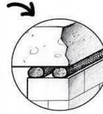
Cordão duplo em cabeça de alvenaria.
