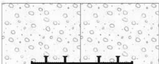
Perfis para estanquidade de juntas de construção externas.
