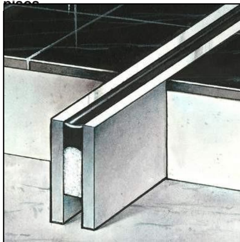
Cantoneiras em alumínio, latão ou inox + elastômero.
