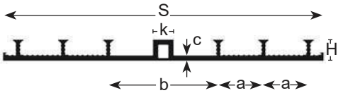
Perfis para estanquidade de juntas de dilatação de superfície.
